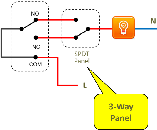
3-Way Wiring
